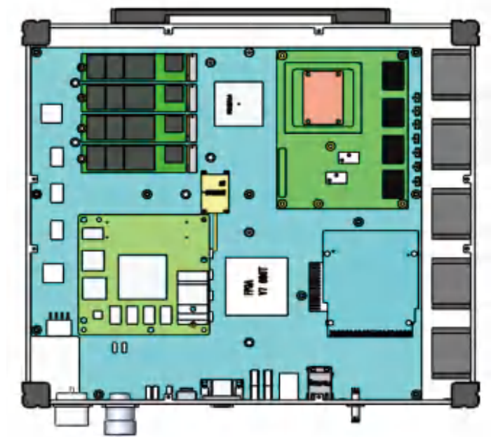
图1 设备的内部组成
